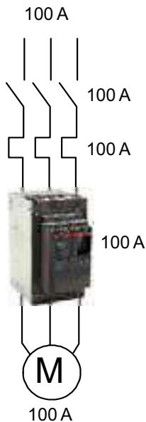
Система плавного пуска, включенная в линию мотора
