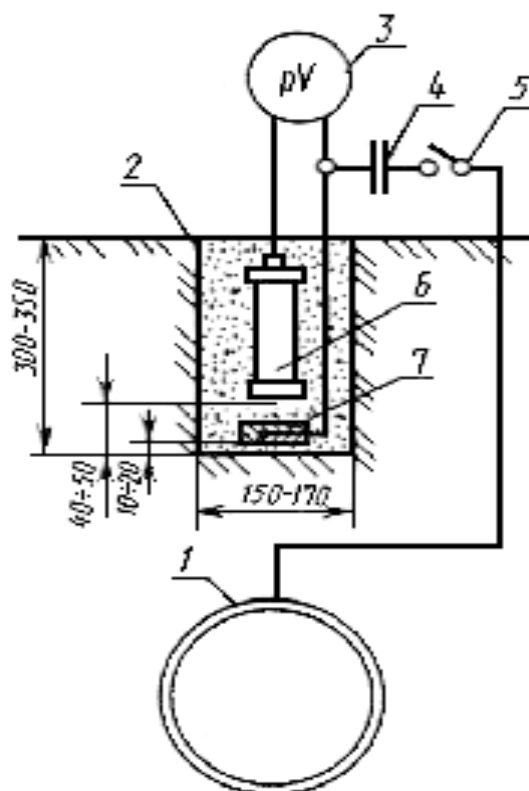
Рисунок 2.6 – Схема измерений смещения потенциала трубопровода: 1 – стальной трубопровод; 2 – шурф; 3 – вольтметр; 4 – конденсатор; 5 – выключатель; 6 – медносульфатный электрод сравнения; 7 – вспомогательный электрод
