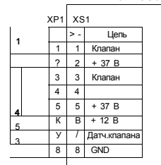
Схема подключения клапана типа КЗЭУГ
