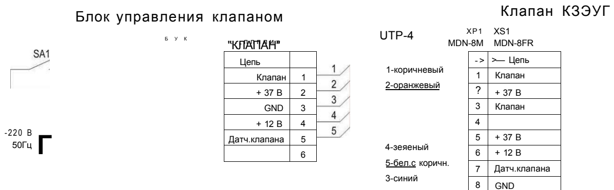
Типовая схема подключения клапана КЗЭУГ к блоку управления клапаном
