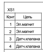
Схема подключения клапана типа КПЭГ (для исполнения БСУ с отключением К1 по второму порогу)
