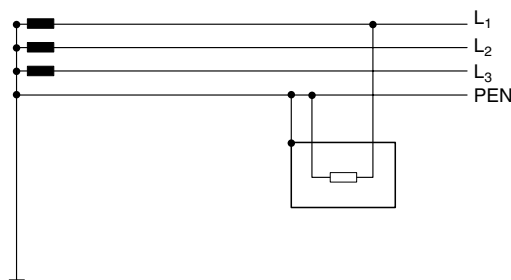
Рисунок 4: система TN-C
