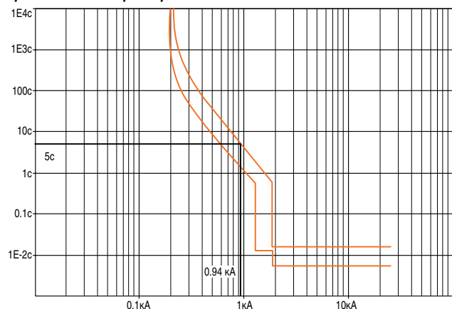
Время-токовая характеристика Tmax XT1C160 In160
