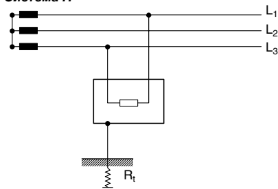
Рисунок 7: Система IT
