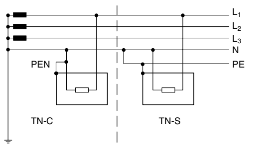
Рисунок 5: система TN-C-S
