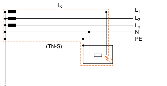
Рисунок 6: замыкание на землю в системе TN
