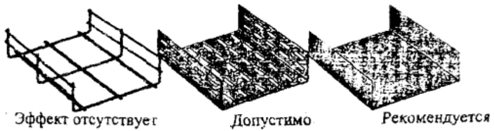
Рис. 21. Влияние конструкции металлических лотков на уровень электромагнитной совместимости
