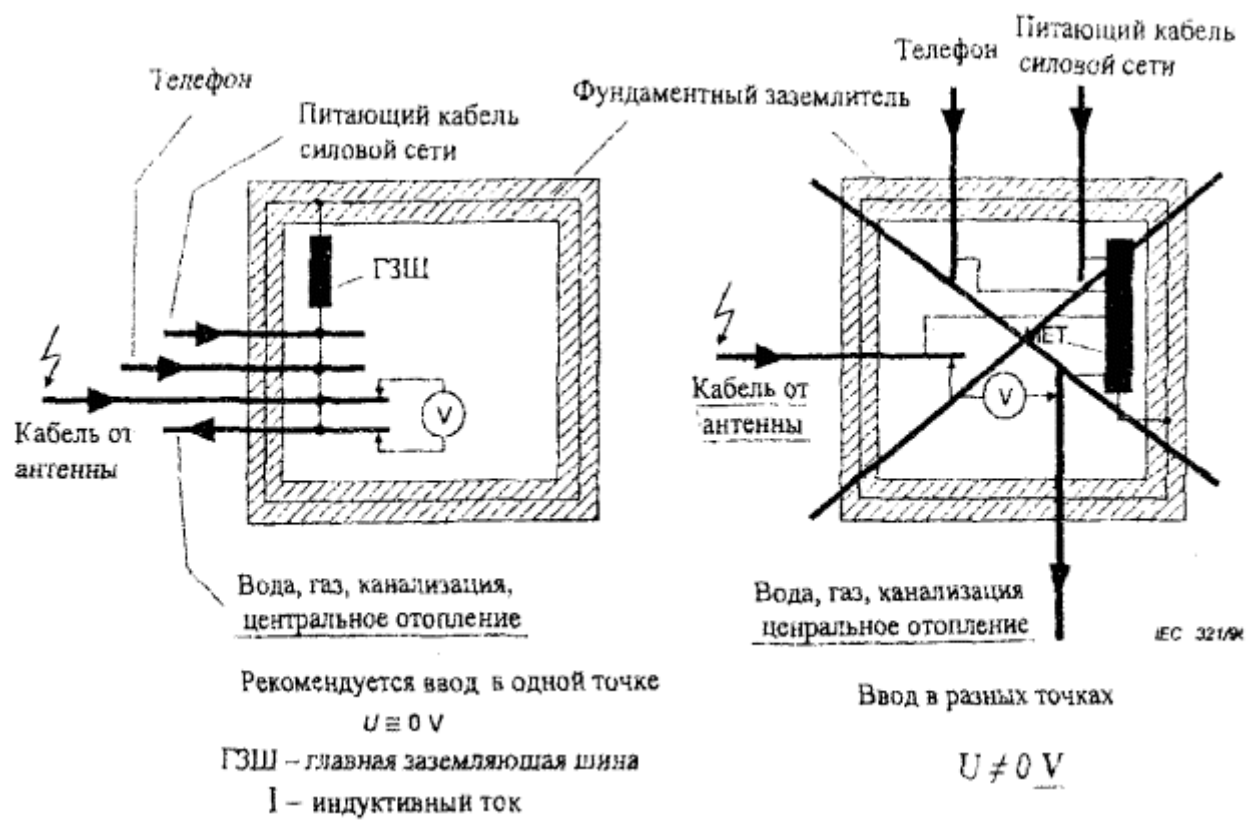
Рис. 9. Примеры ввода в здание бронированных кабелей и металлических труб
