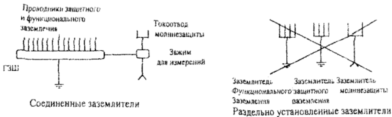
Рис. 12. Соединение заземлителей.
