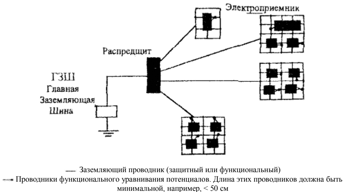
Рис. 14. Пример радиально-сетчатой системы уравнивания потенциалов
