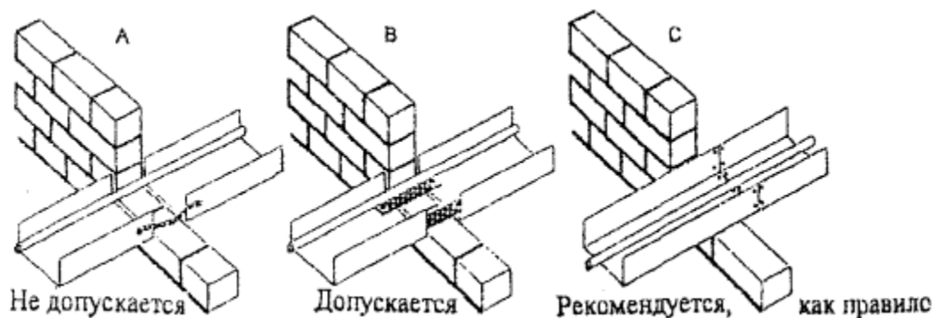
Рис 25. Соединение секций металлических лотков в местах прохода сквозь стену
