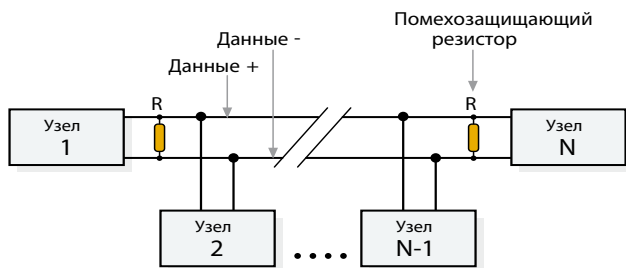
Рис. 14. Многоточечная система с шиной RS-485
