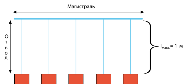
Рис. 23а. Сеть с топологией «шина» («шлейф»)
