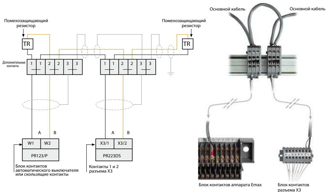
Рис. 23. Схема подключения автоматических выключателей Emax и Tmax к коммуникационной сети Modbus
