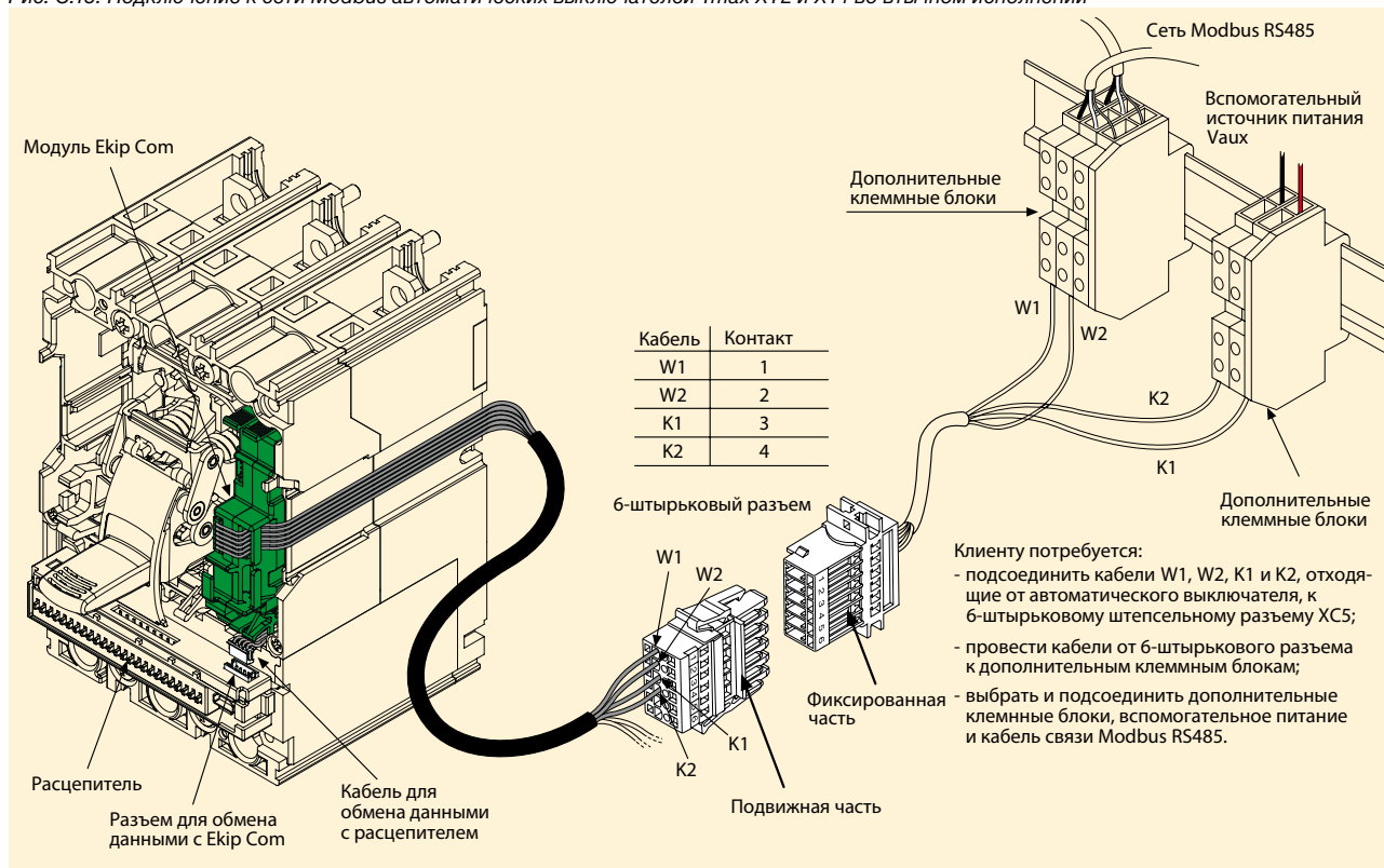
Рис. С.13. Подключение к сети Modbus автоматических выключателей Tmax XT2 и XT4 во втычном исполнении
