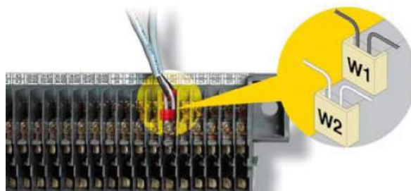
Рис. 26. Подключение главного кабеля прямо к зажимам блока контактов выключателя
