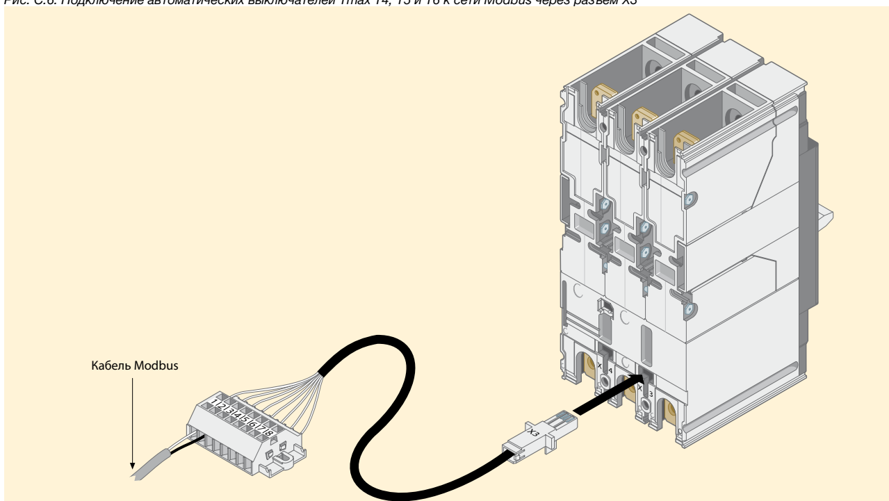
Рис. С.6. Подключение автоматических выключателей Tmax T4, T5 и T6 к сети Modbus через разъем X3
