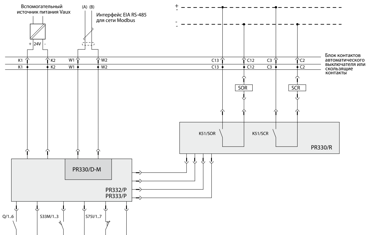
Рис. С.3. Схема подключения PR33X/P к сети Modbus по модулю PR330/D-M
