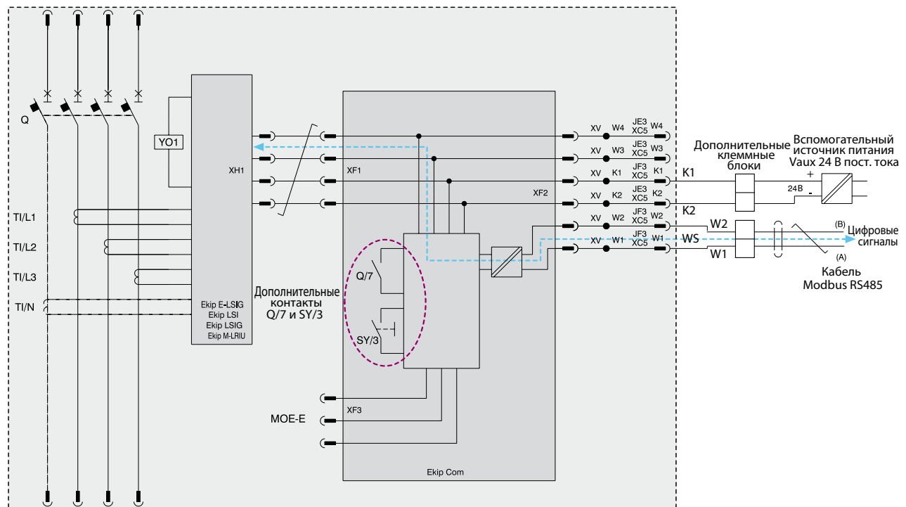
Рис. С.8. Схема электрического подключения к сети Modbus расцепителей Ekip E-LSIG, Ekip LSI, Ekip LSIG и Ekip M-LRIU с модулем Ekip Com. Автоматический выключатель в выкатном исполнении.
