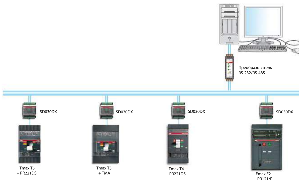
Рис. 19. Интерфейсный модуль SD030DX
