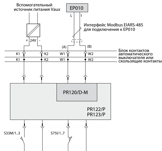
Рис. С.2. Схема подключения расцепителей PR122/P-PR123/P к модулю EP010
