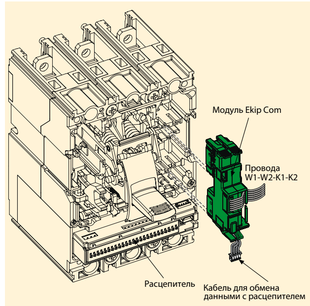
Рис. С.12. Подключение к сети Modbus стационарных автоматических выключателей Tmax XT2 и XT4
