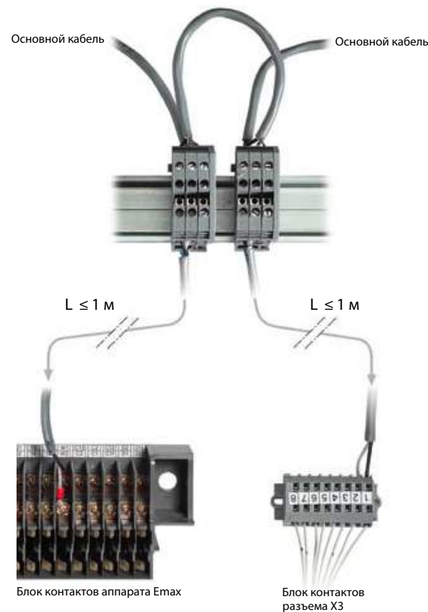
Рис. 27. Подключение к блоку контактов выключателя через дополнительный клеммный блок
