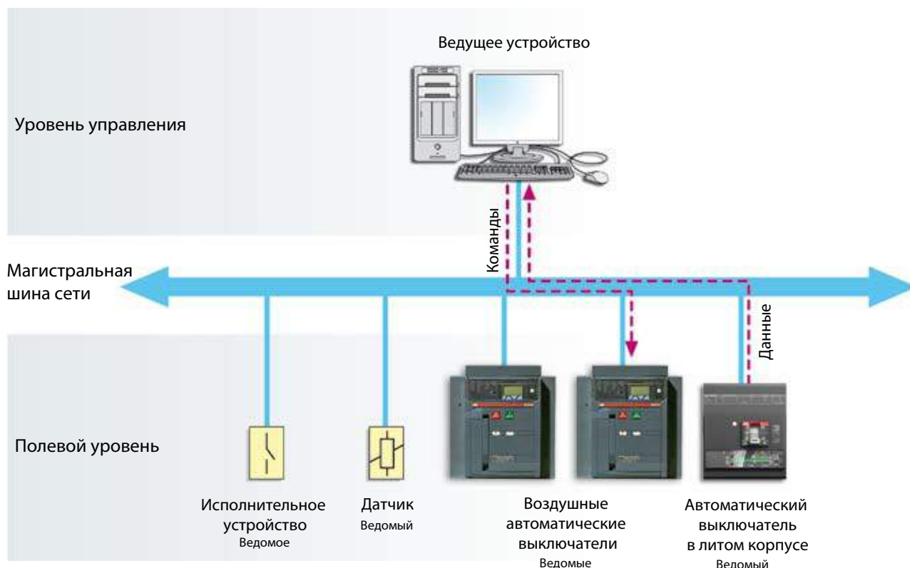
Рис. 17. Система управления с двухурвневой архитектурой
