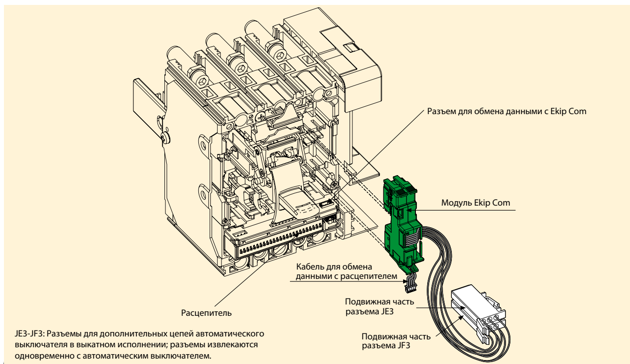
Рис. С.10. Подключение к сети Modbus автоматических выключателей Tmax XT2 и XT4 в выкатном исполнении
