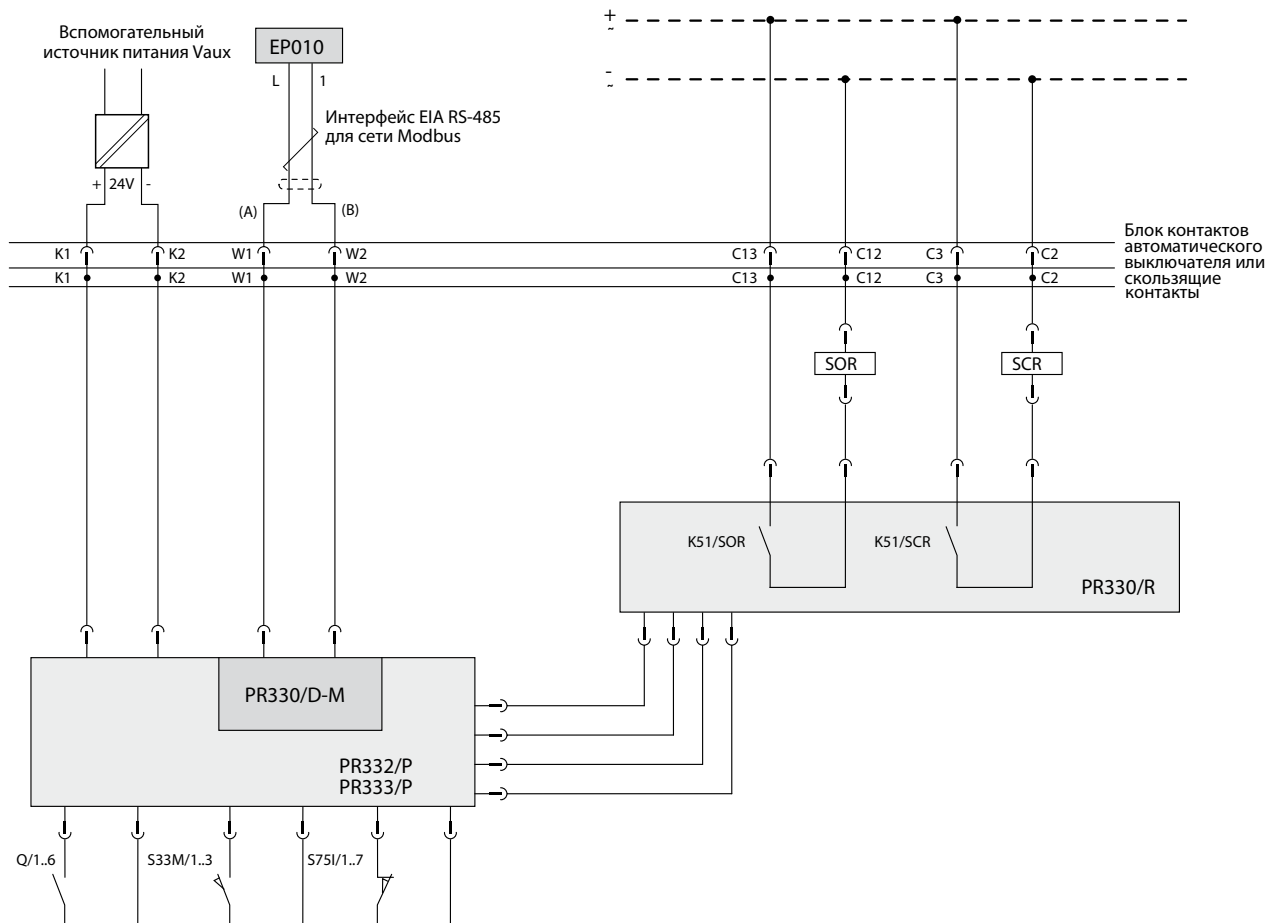
Рис. С.4. Схема подключения PR33X/P к модулю EP010
