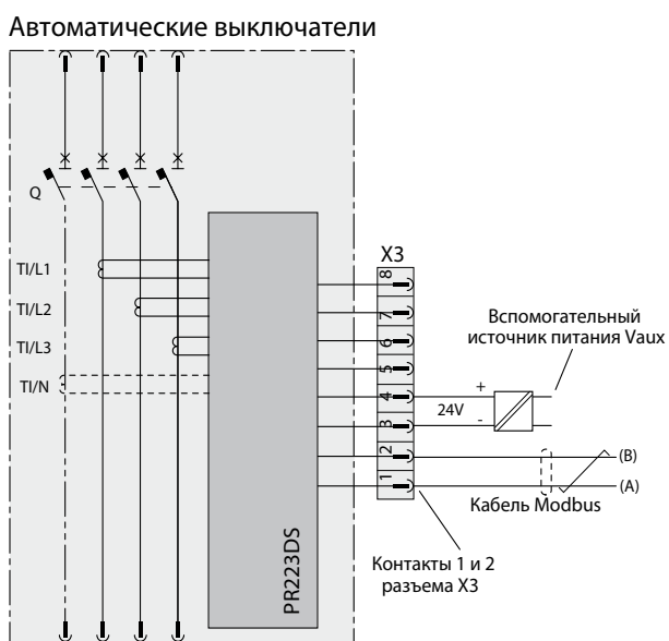
Рис. С.6. Подключение автоматических выключателей Tmax T4, T5 и T6 к сети Modbus через разъем X3
