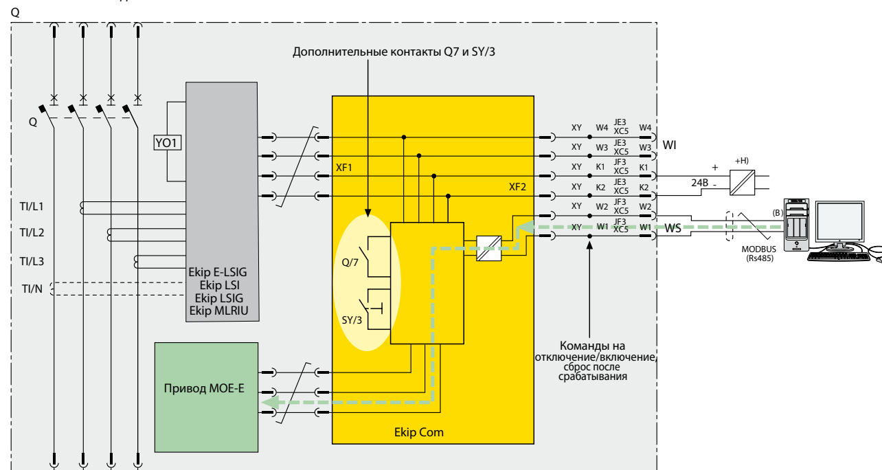
Рис. F.1. Схема соединения с МОЕ-Е
