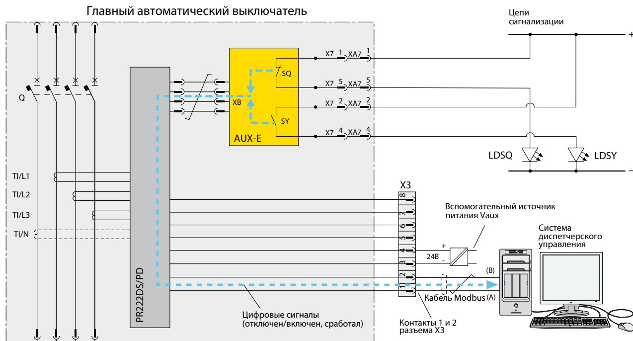
Рис. Е.2. Схема соединений контактов AUX-E, подключенных к PR222DS/PD
