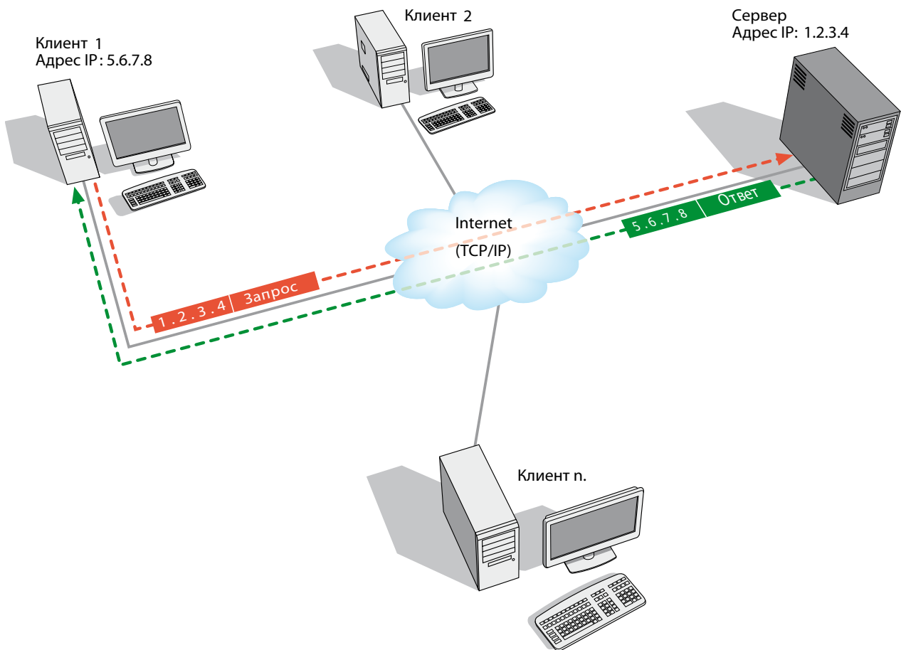
Рис. 37. Последовательность запрос/ответ
