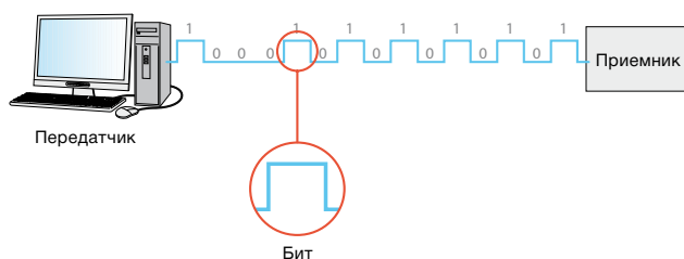
Рис. 1. Последовательность битов
