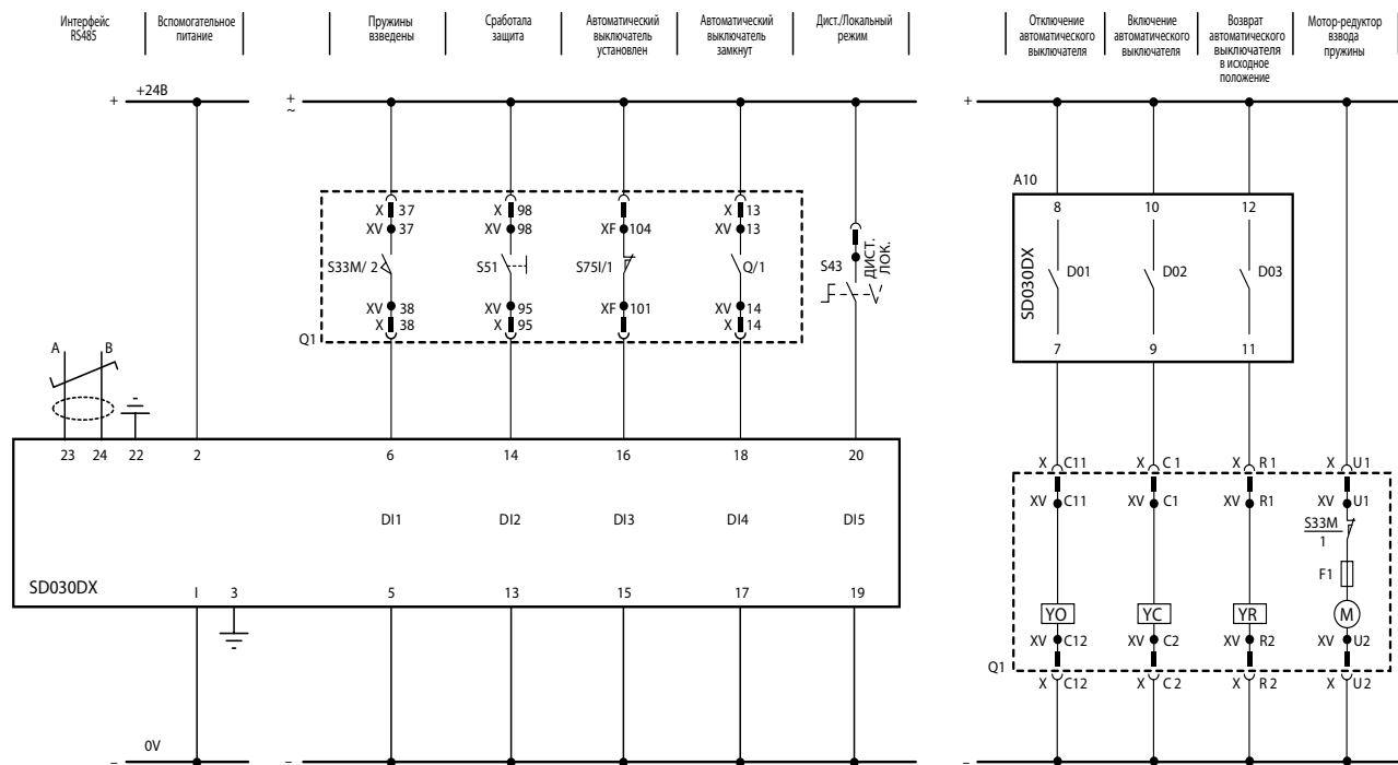
Рис. 21. Схема соединений SD030DX для автоматического выключателя Emax E6
