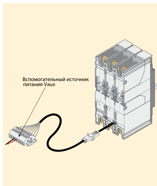
Рис. В.2. Вспомогательный источник питания для автоматических выключателей в литом корпусе T4, T5 и T6
