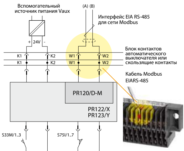
Рис. С.1. Схема подключения PR12X/P/DC к сети Modbus по модулю PR120/D-M
