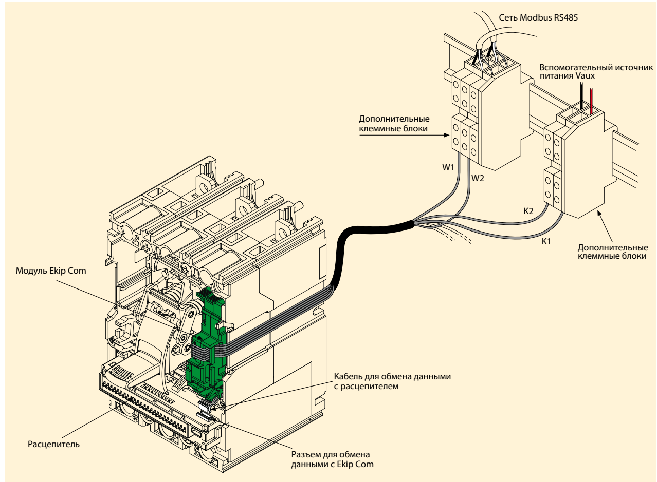
Рис. С.12. Подключение к сети Modbus стационарных автоматических выключателей Tmax XT2 и XT4
