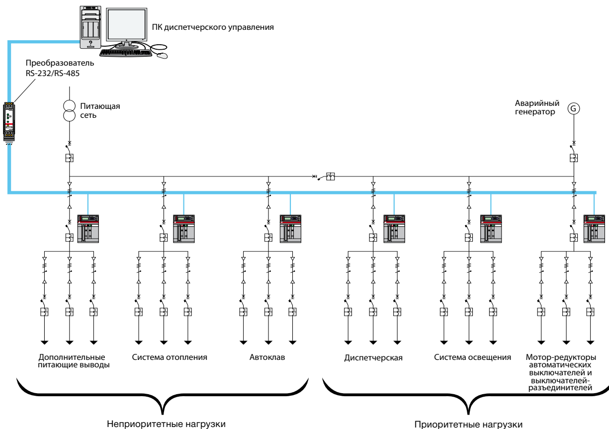
Рис. 41. Схема питания служб жизнеобеспечения электростанции, получаемой от вспомогательных систем
