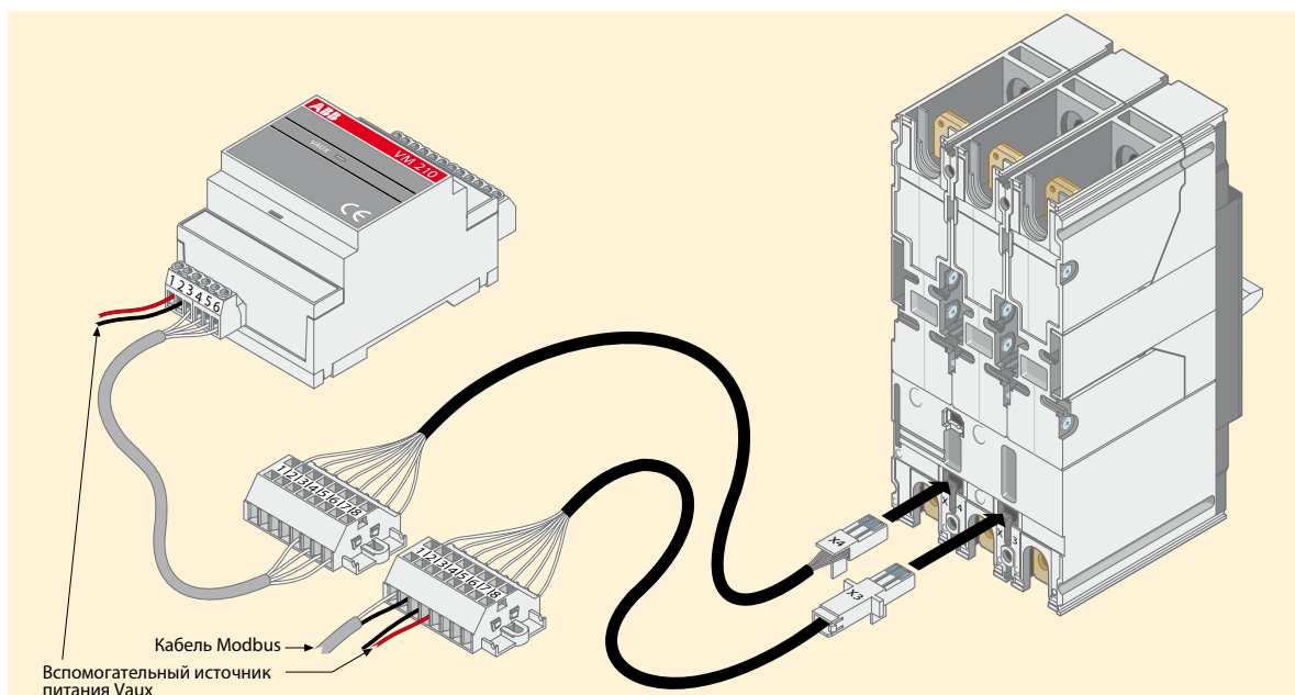
Рис. D.5. Подключение модуля VM210 к разъему X4
