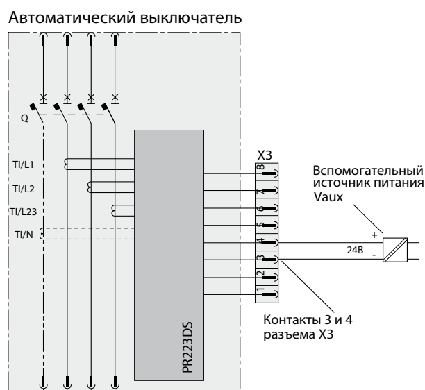
Рис. В.1. Схема подключения вспомогательного источника питания для расцепителя P223DS.
