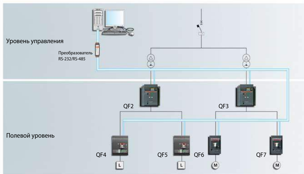
Рис. 32. Система диспетчерского управления и контроля распределительной электроустановки низкого напряжения
