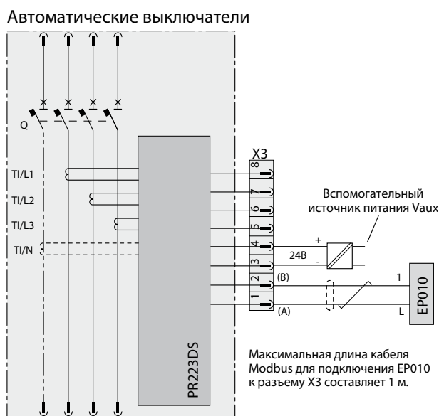
Рис. С.7. Схема подключения модуля EP010 автоматического выключателя Tmax
