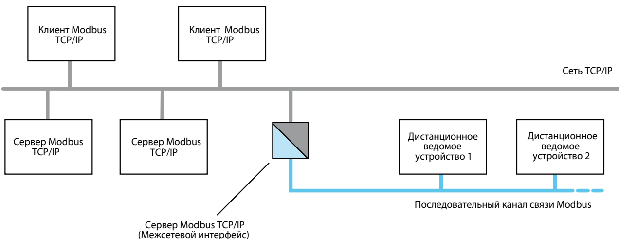
Рис. 36. Сеть Ethernet TCP/IP – Последовательный канал связи Modbus
