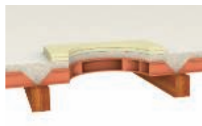
Балочное перекрытие
