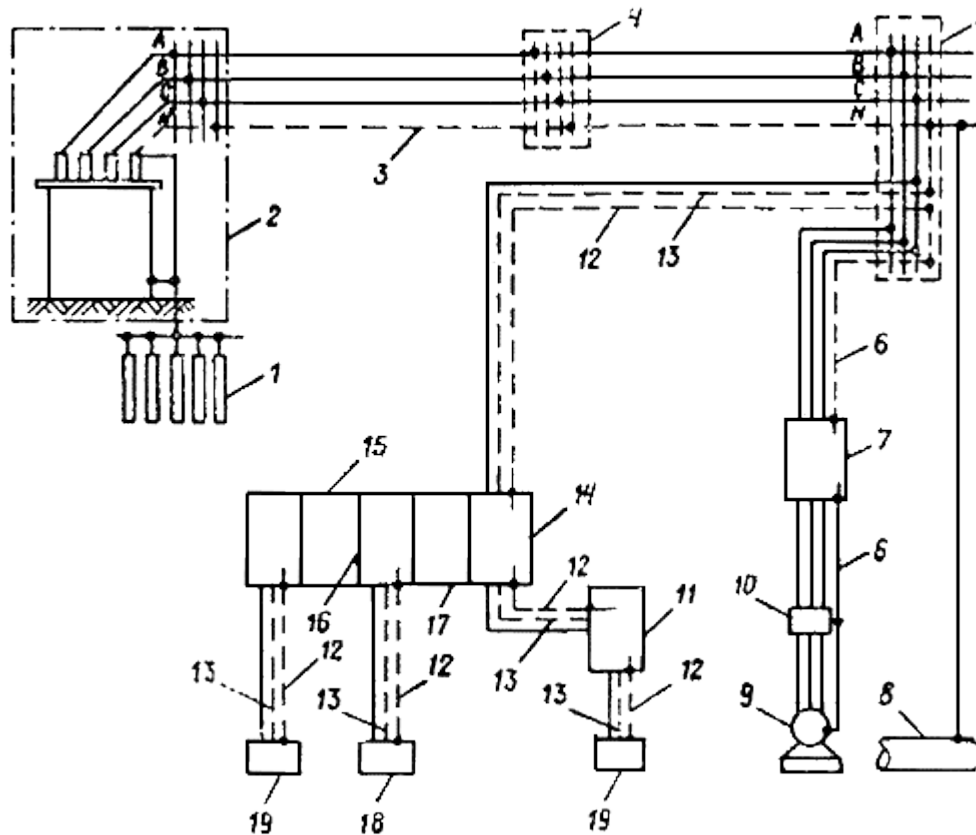
Рис.3. Пример выполнения зануления в электроустановке системы автоматизации:
