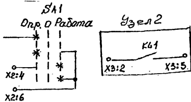
Рис.1 Электрическая принципиальная схема управления перевертышкой электроприводом насоса маслобака для режимов "Опробование" и "Работа".
